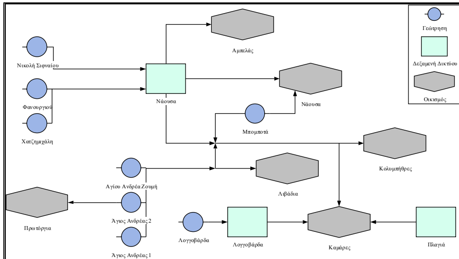
Σχήμα 7.4-2: Δίκτυο Ύδρευσης Δ.Δ. Νάουσας (Δ.Ε.Υ.Α.Π, 2001)
